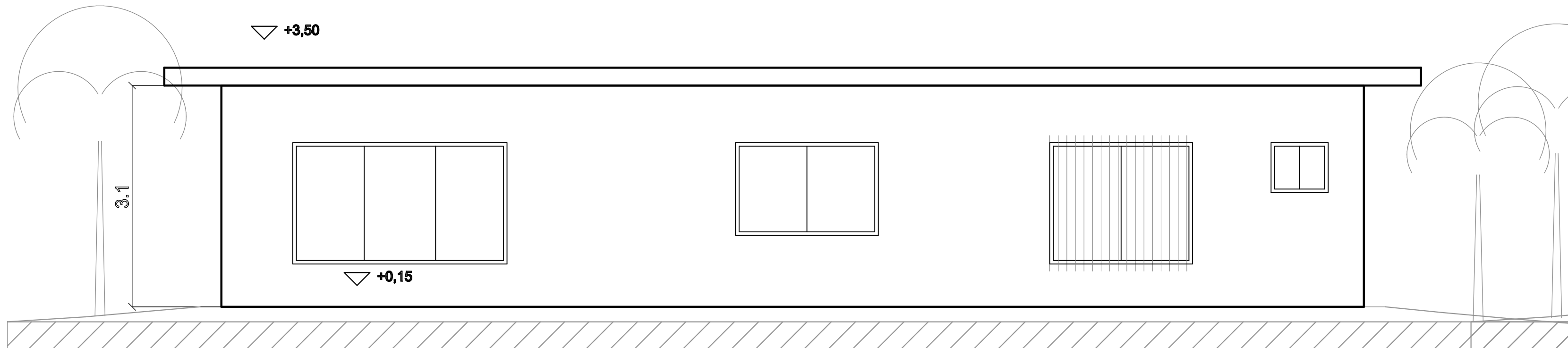
ELEVAÇÃO NORTE ESCALA 1:50
