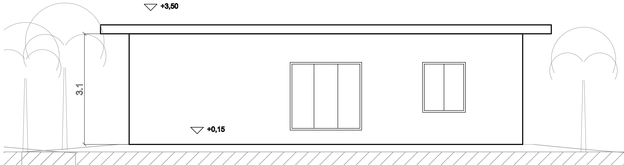
ELEVAÇÃO LESTE ESCALA 1:50
